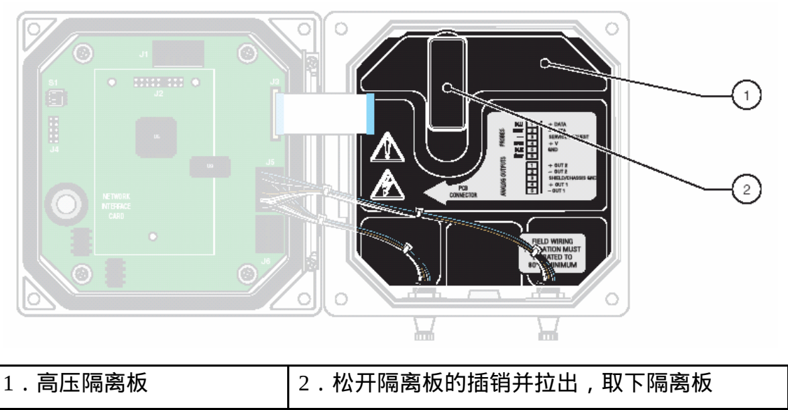
图 3-11 去掉高压隔离板
